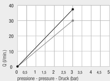
Diagramma di portata Flow diagram Diagramm der Durchflussleistung
