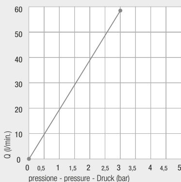
Diagramma di portata Flow diagram Diagramm der Durchflussleistung
