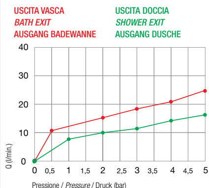
Diagramma di portata (uscita libera) Flow diagram (free exit) Diagramm der Durchflussleistung (freier Ausgang)
